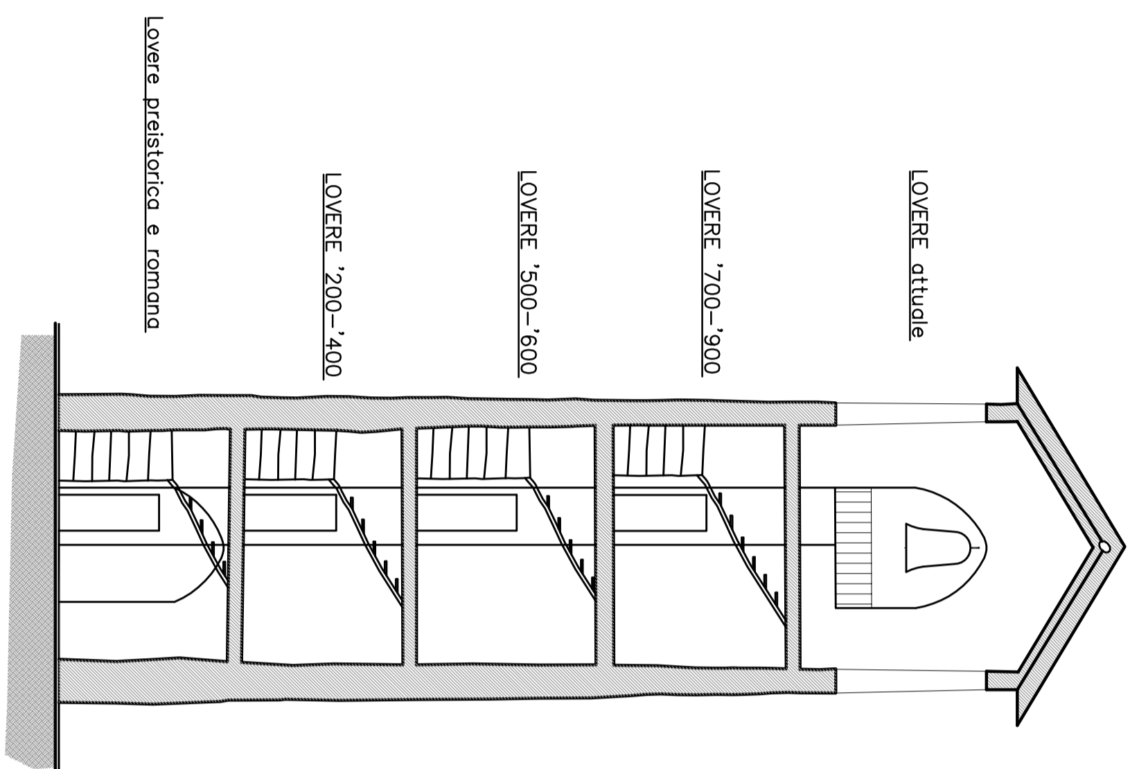
SEZIONE TIPO TORRE CIVICA DI LOVERE sintesi della storia cittadina
