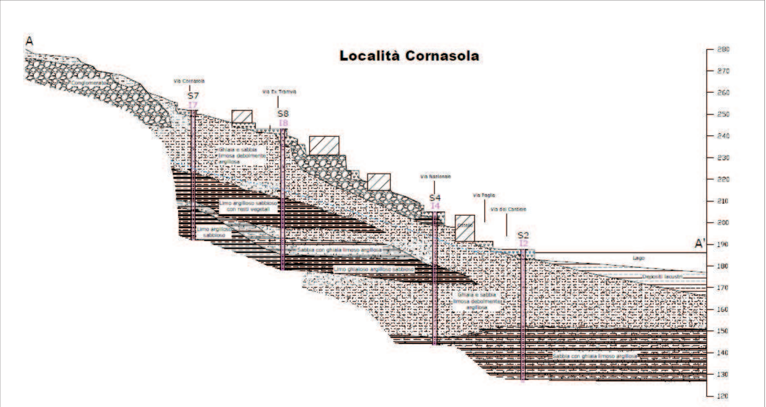
(Sezione tratta da "Rapporto sulle indagini geognostiche loc. Cornasola" a firma dott. Feriti e dott. Sigala - Luglio 2016)
